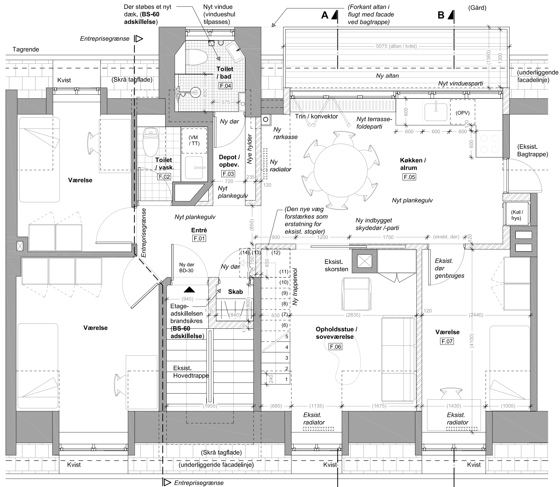
5. SAL / TAGETAGE - FREMTIDIGE FORHOLD - MÅL 1:50
