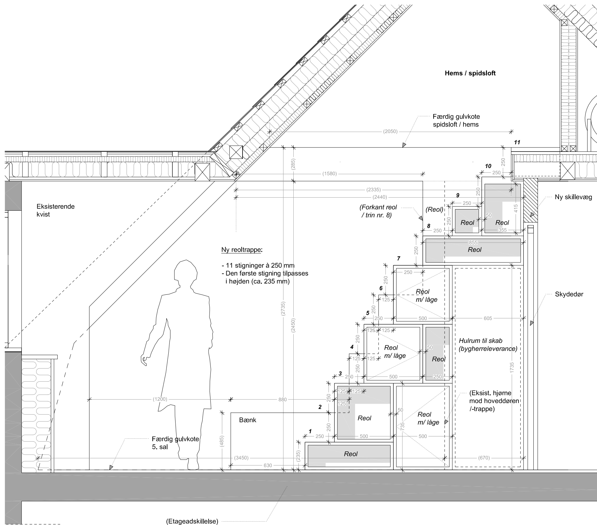
SIDEOPSTALT - MÅL 1:20
